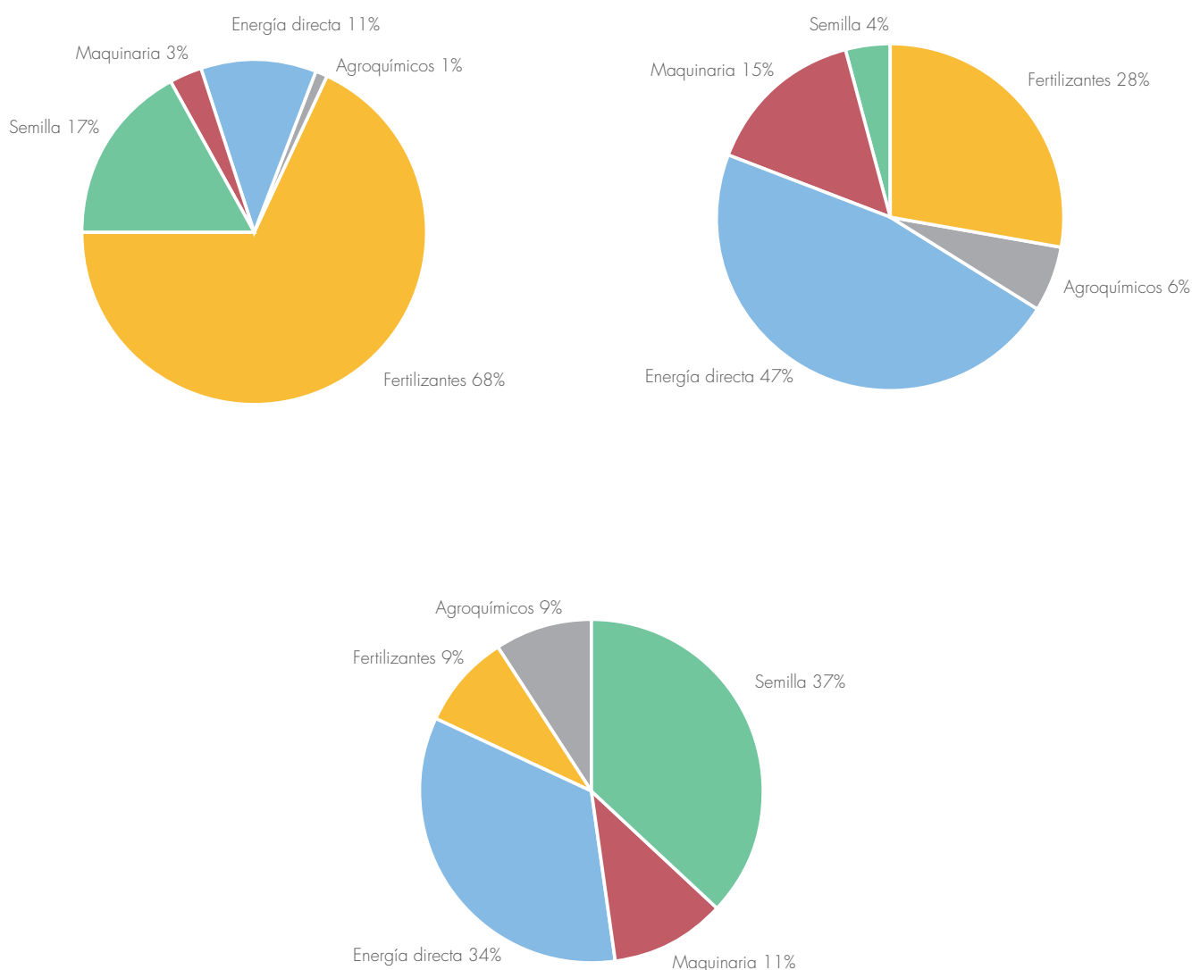
Figura 21. Consumo medio de energía por cultivo y sistema de manejo
