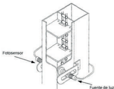
Figura 30. Sistema de medida de rendimiento mediante fotosensores que miden el volumen de grano que pasa instantáneamente
