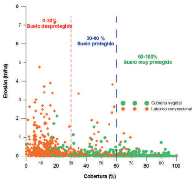
Figura 7. Erosión del suelo en función del porcentaje de superficie cubierta por restos vegetales. Fuente: AEAC.SV.
